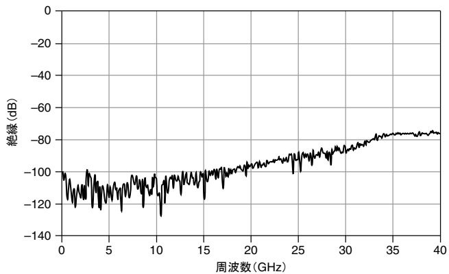
図 2. 標準絶縁
