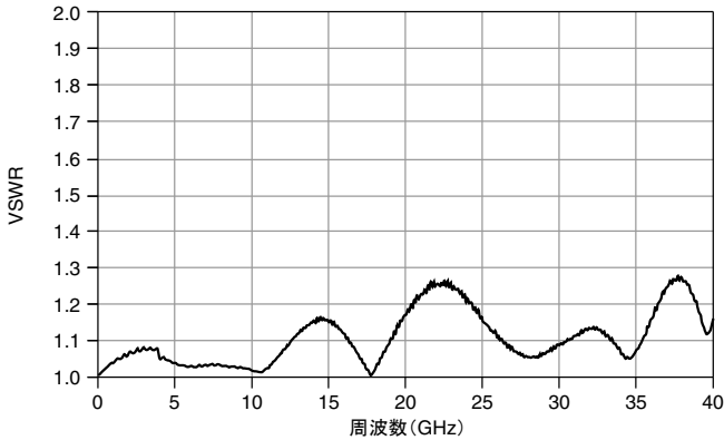
図 3. 標準 VSWR
